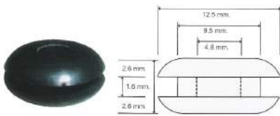
ยางกันบาดทะลุ
